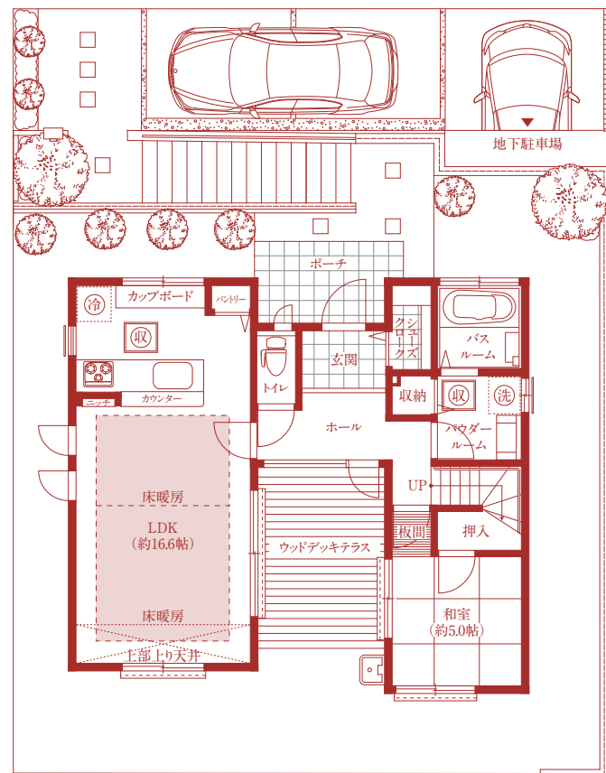
1階平面図
